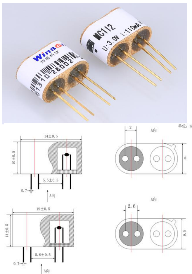
图 1：传感器外形结构图
