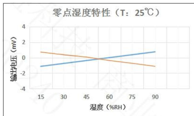
图 7: 零点湿度特性曲线
