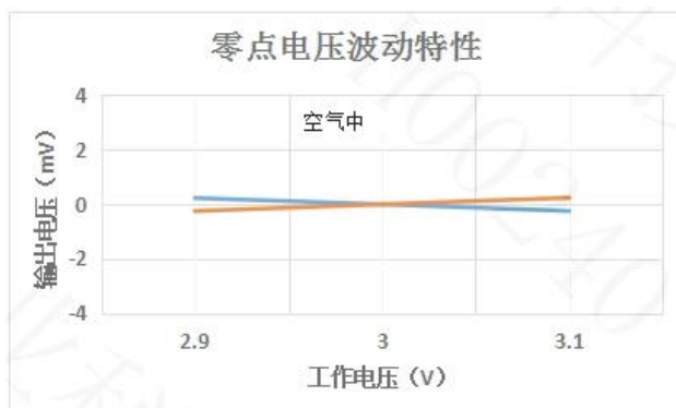
图9: 零点电源波动特性曲线
