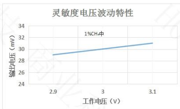
图10: 灵敏度电源波动特性曲线
