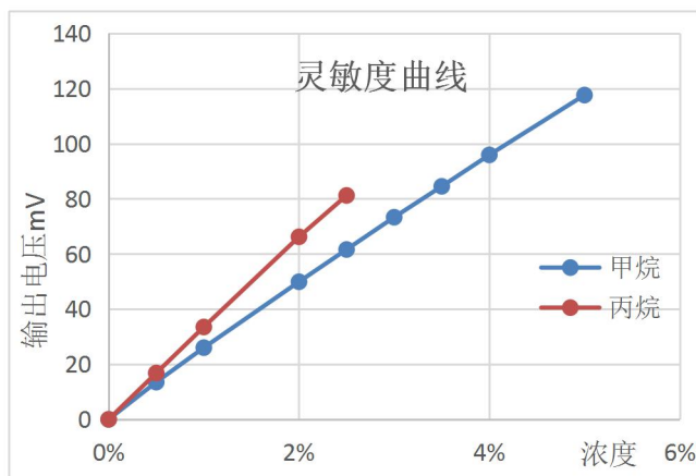
图 3: 灵敏度曲线
